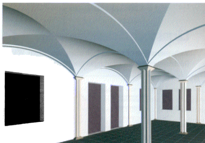
Projekt Stadthaus-Atelier, Zweisäulenraum, Modell Florenz, mit Säulenmodell Passau
